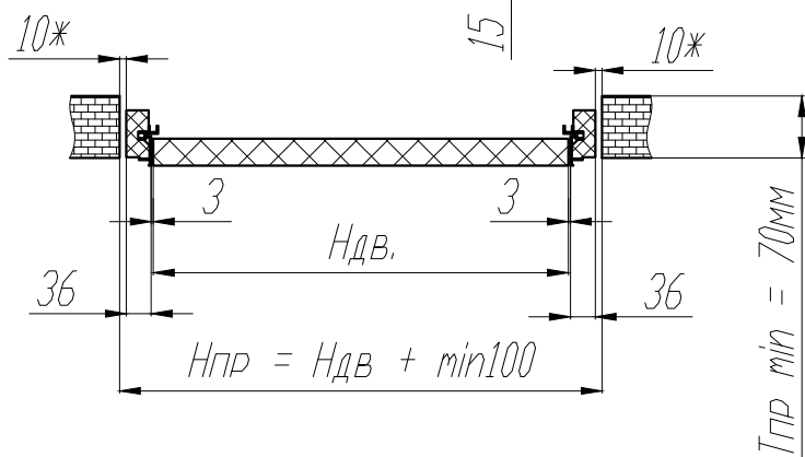
Рис. 2. Расчет проема для скрытых полотен
