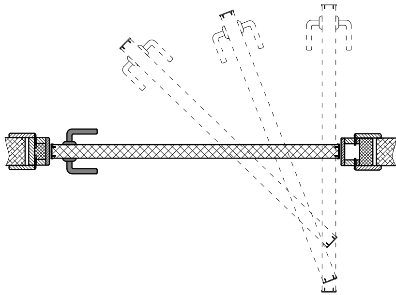
Рото механизм (правое открывание от себя)
