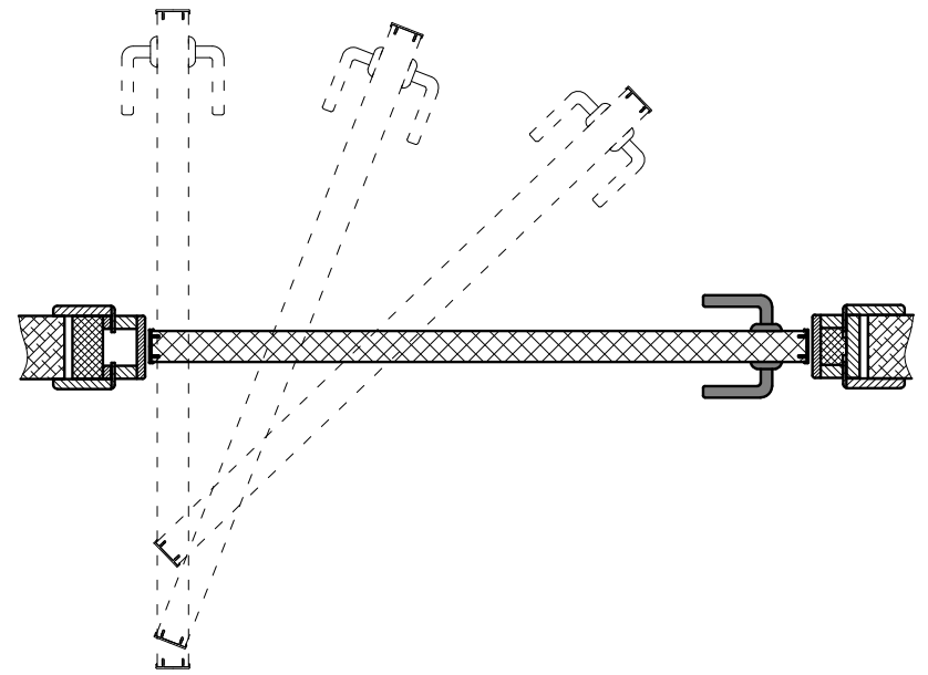
Рото механизм (левое открывание от себя)
